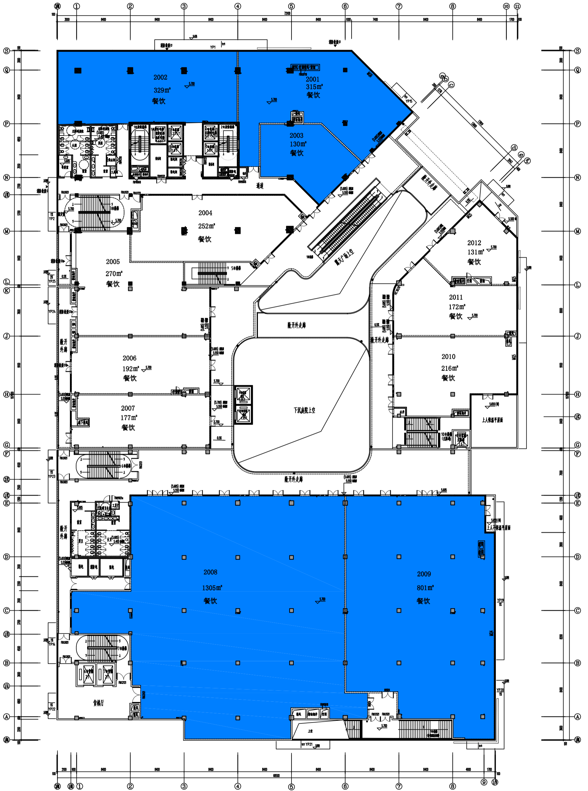
二层平面图
